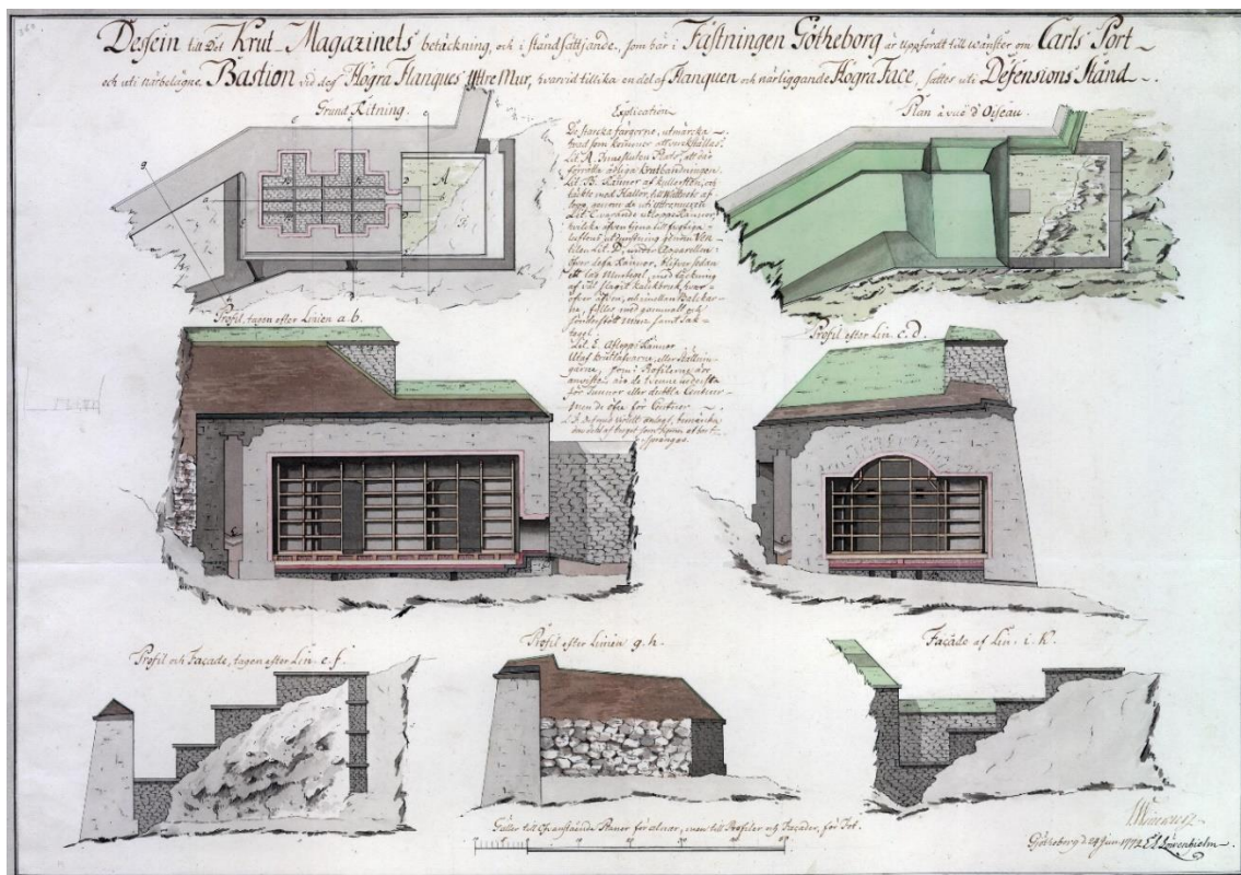
Figur 2 Planritningen, eller så kallad dessein , från 1772 över arbetena vid krutrummet som planerades att färdigställas det året. Krigsakrivet SFP Göteborg 239.
